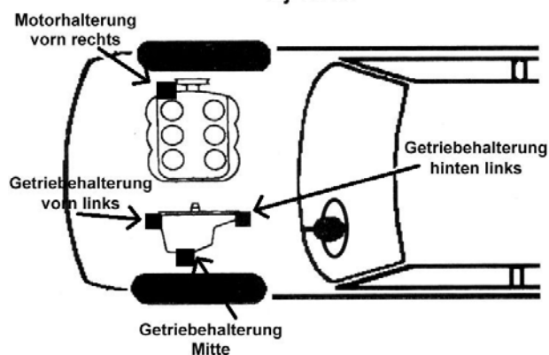
Positionen der Motor- und Getriebehalterungen
