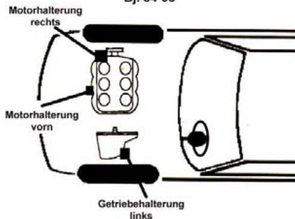
Positionen der Motor- und Getriebehalterungen
